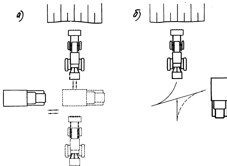
Рис. 12. Схема работы погрузчика
