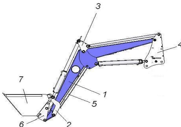
Рис.8 Подъемное устройство 1-рама подъема, 2- кронштейн, 3- кронштейн, 4- кронштейн, 5- опора, 6- переходник, 7-ковш
